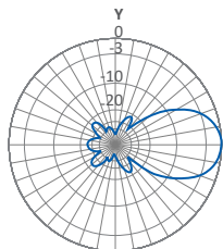
DIAGRAMA DE RADIACIÓN
