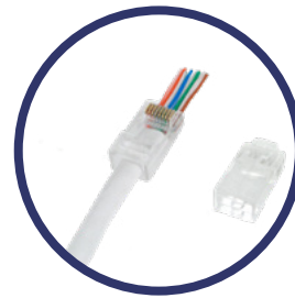
Detalle montaje
